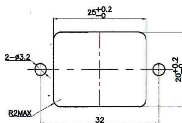
取付穴参考图
