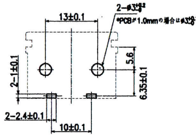
基板取付穴参考寸法
