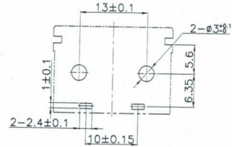
刻印配置图 1.5:1
