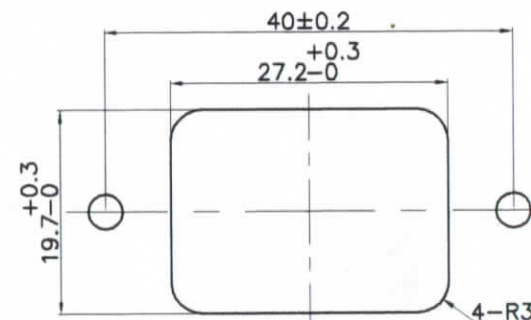
取付穴参考图
