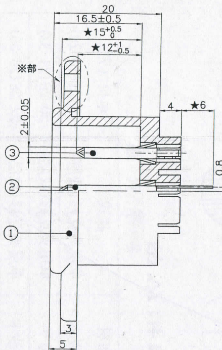
SEC A-A
