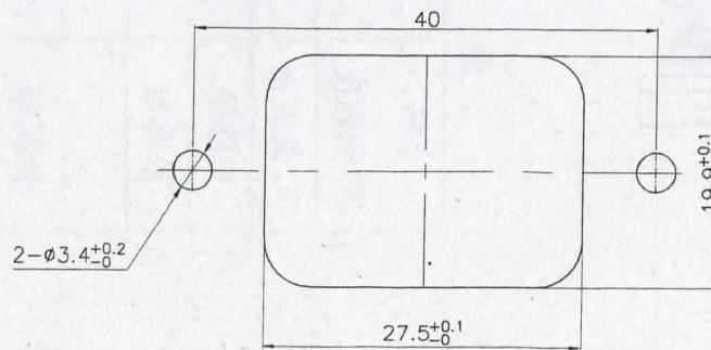
取付穴参考图
