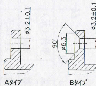
※部详细图
