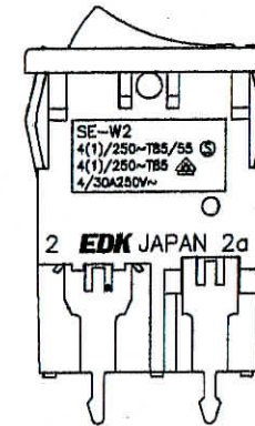
本体取付穴参考図
