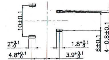
PCB取付穴参考図
