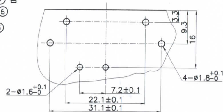
PCB板参考图
